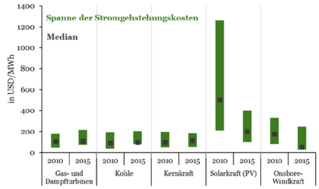
Quelle: Prognostizierte Stromgestehungskosten der IEA und NEA (2015), ETF Securities.
